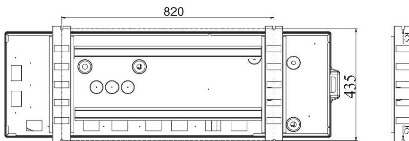
Vista superior
