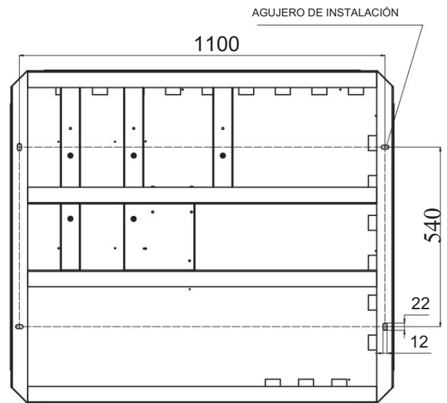
Vista inferior
