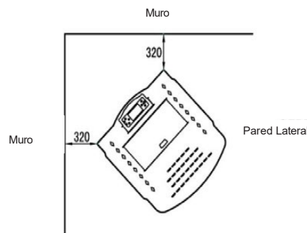
Instalación en esquina
