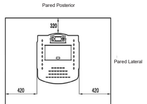
Instalación en paralelo
